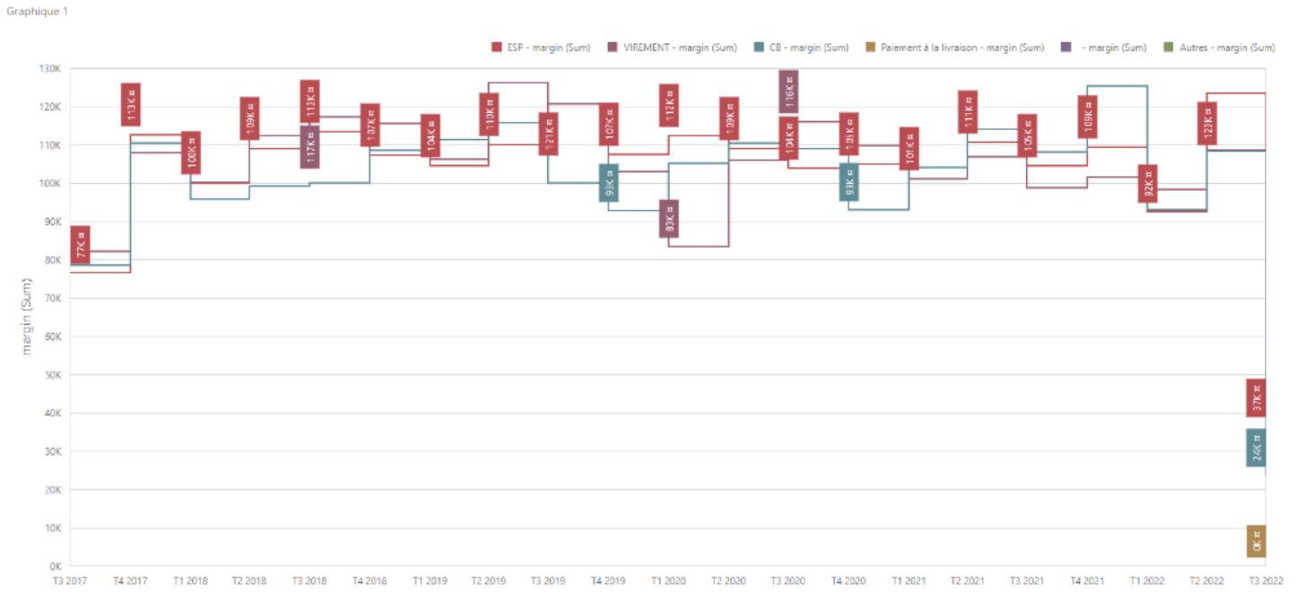
Graphique Spline
