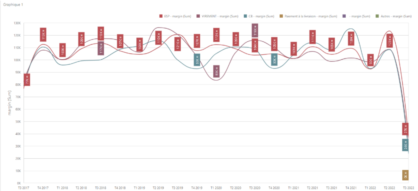
Graphique zone
